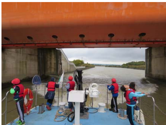
茨戸川から石狩川へ
